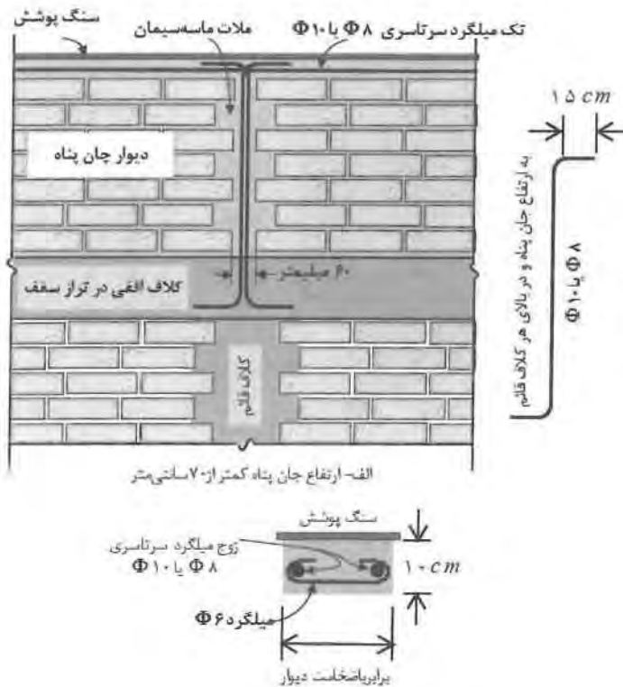
شکل ۷-۱۶ جزئیات مهار جان‌پناه
