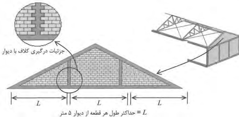
شکل ۷-۲۵ کلاف بندی دیوار انتهایی زیر سقف های شیبدار
