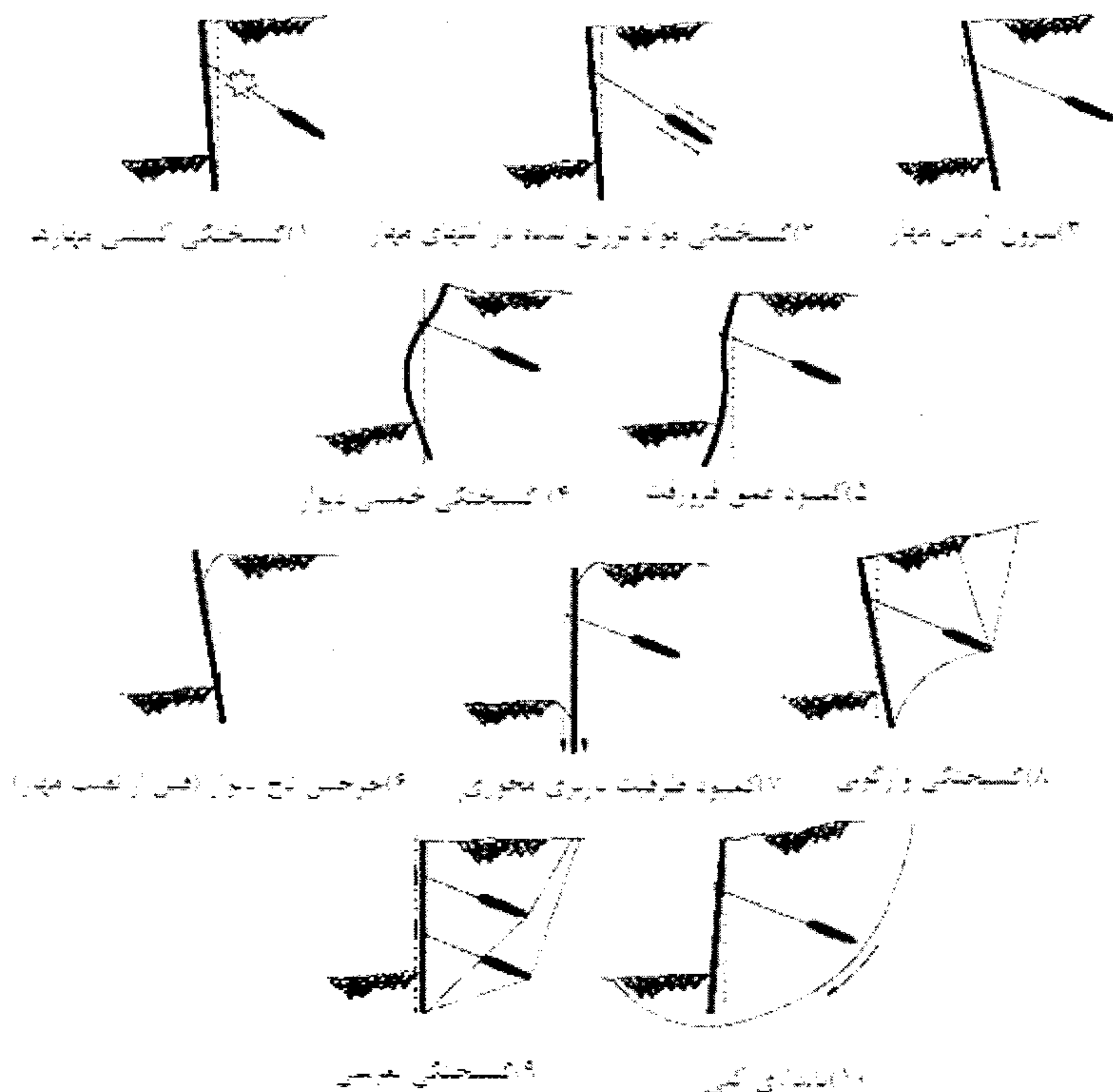
شکل ۷-۵-۱ حالت‌های حدی دیوارهای مهار شده
